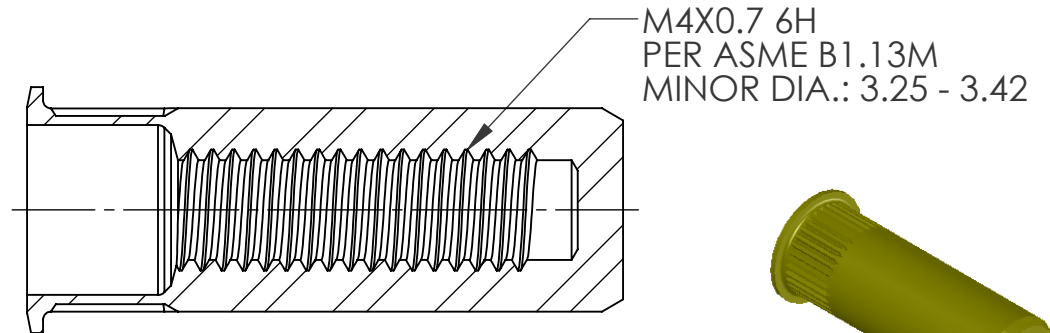
SECTION A-A
