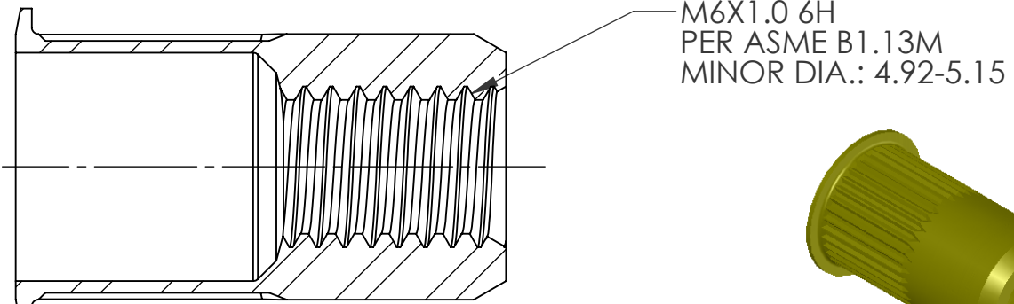
SECTION A-A
