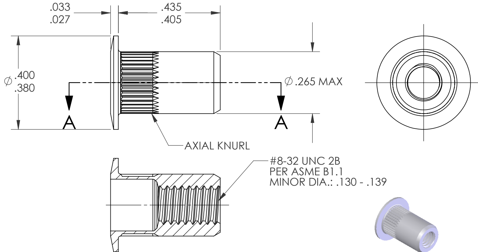
SECTION A-A
