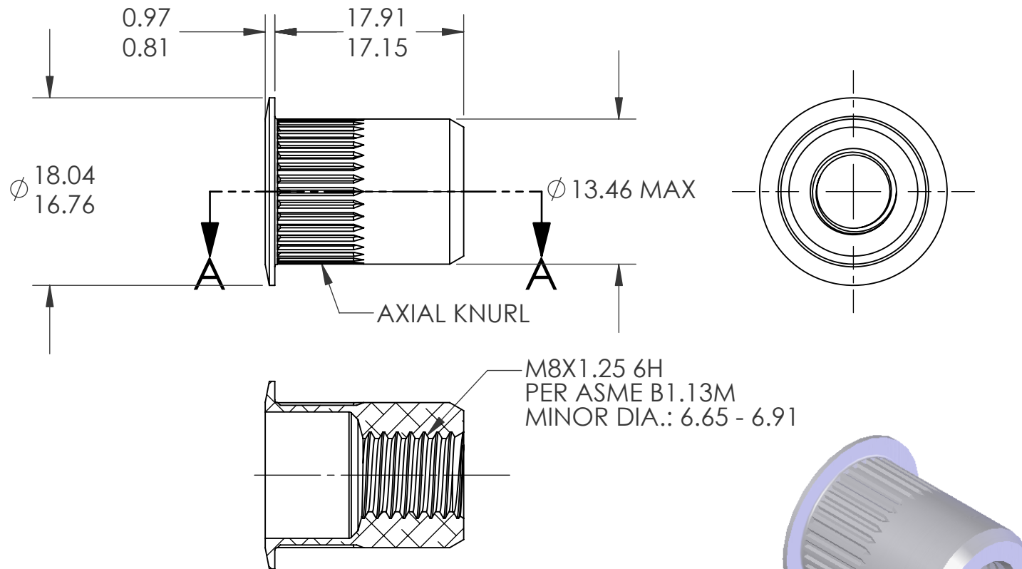
SECTION A-A
