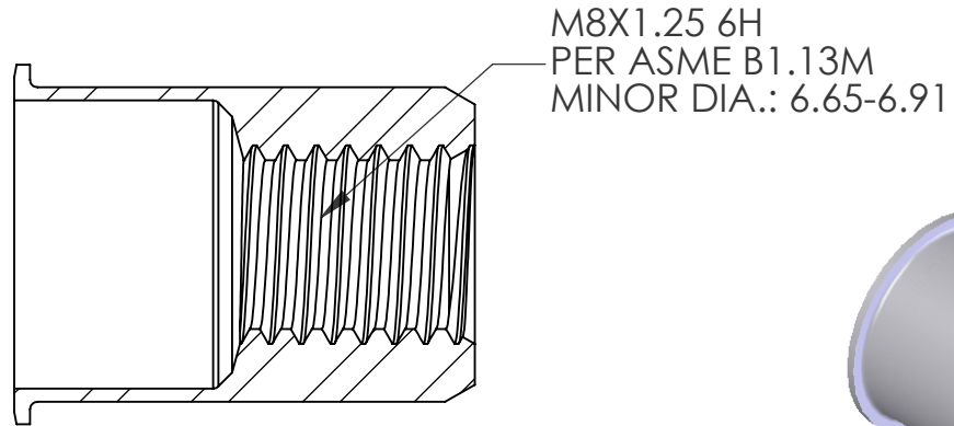
SECTION A-A SCALE 3 : 1
