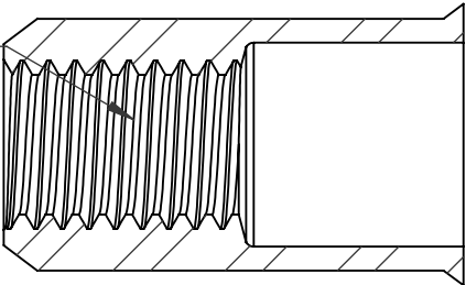
SECTION A-A SCALE 4 : 1
