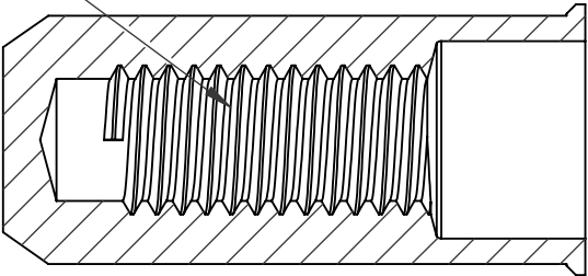
SECTION A-A SCALE 3 : 1
