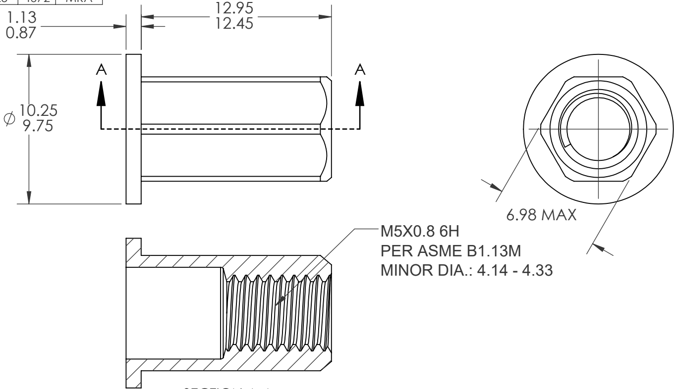
SECTION A-A SCALE 4 : 1
