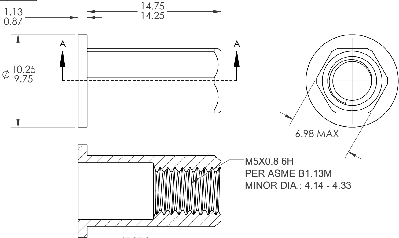
SECTION A-A SCALE 4 : 1
