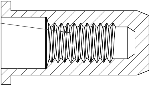
SECTION A-A SCALE 3 : 1
