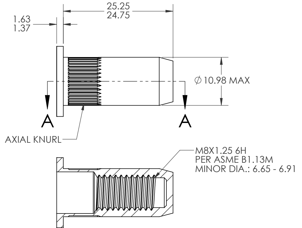
SECTION A-A
