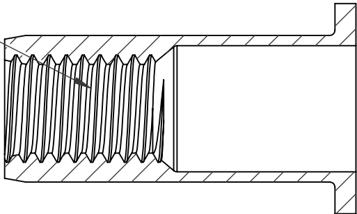
SECTION A-A SCALE 4 : 1
