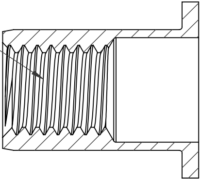
SECTION A-A SCALE 3 : 1
