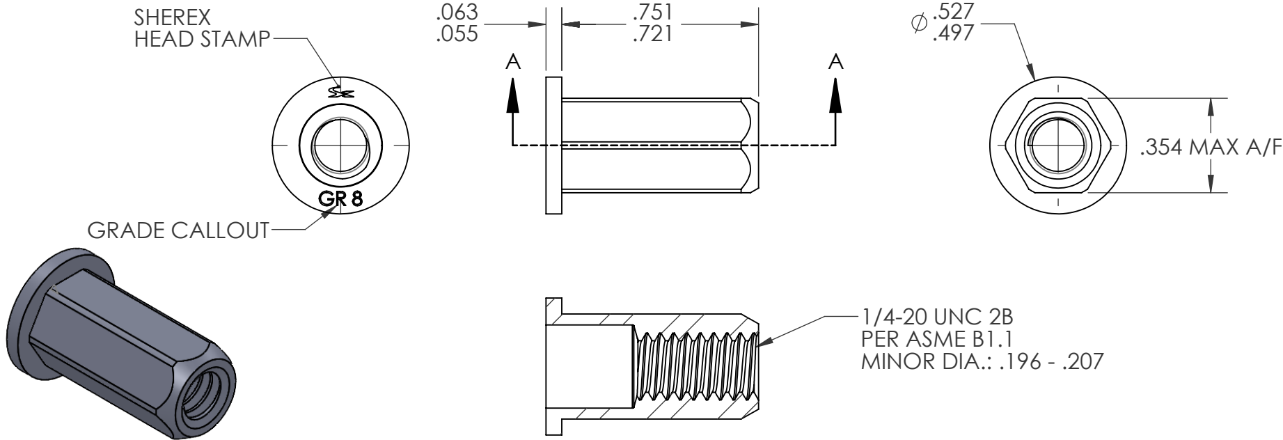
SECTION A-A
