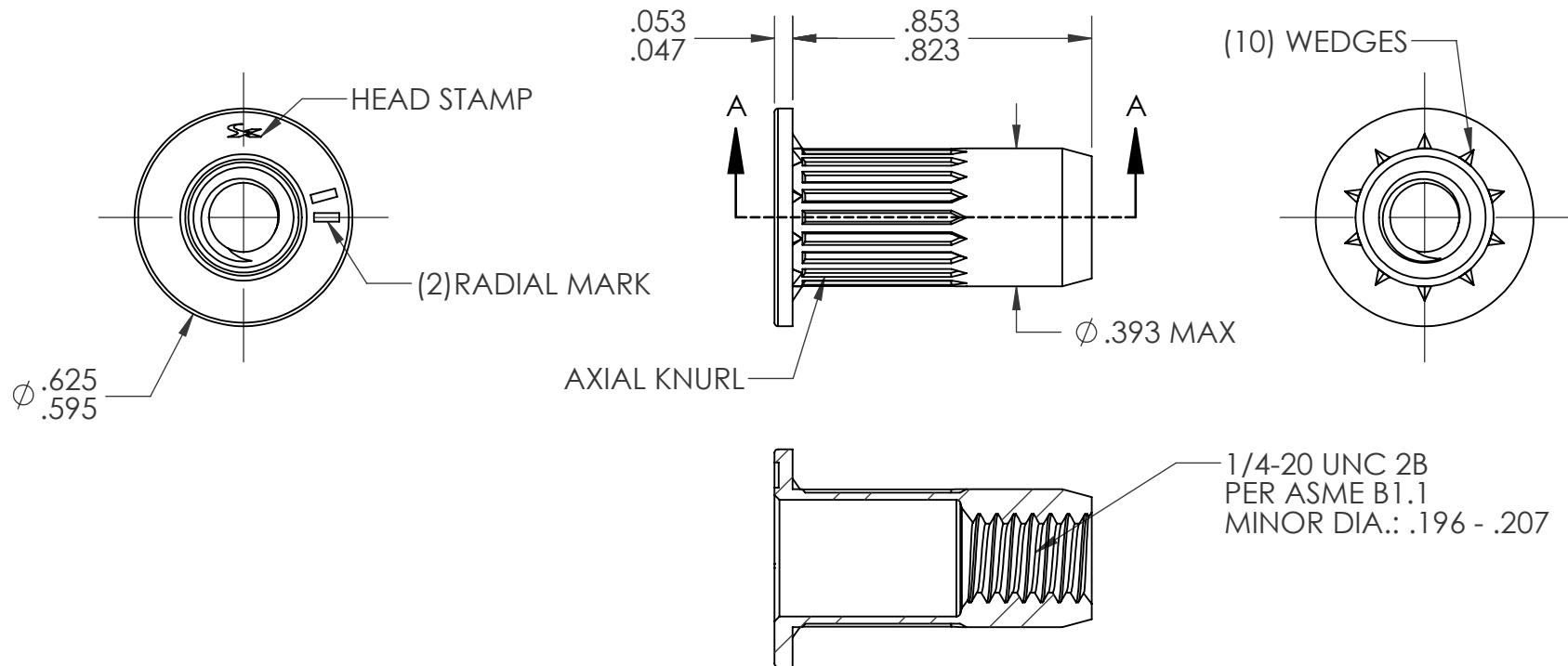
SECTION A-A
