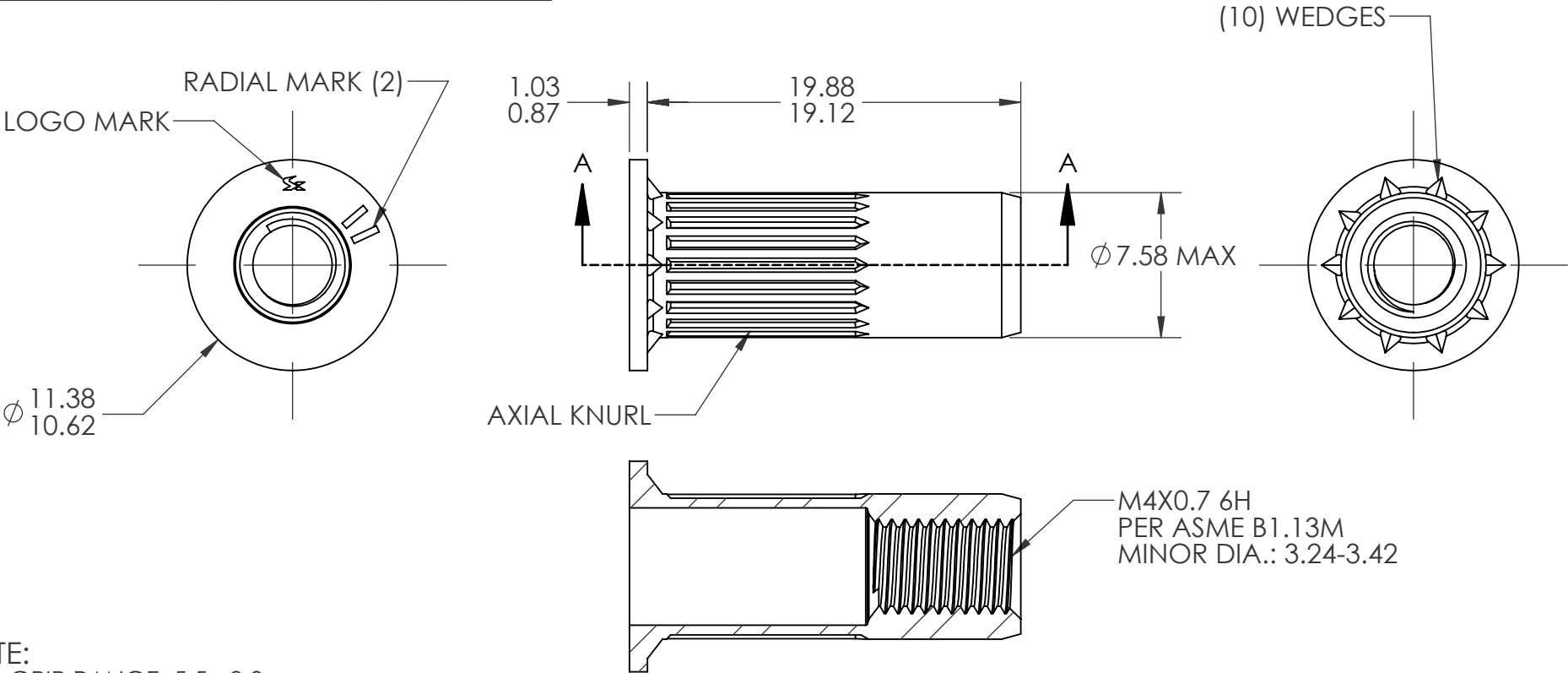
SECTION A-A
