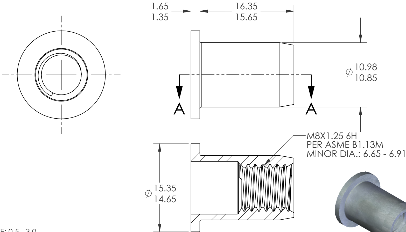
SECTION A-A
