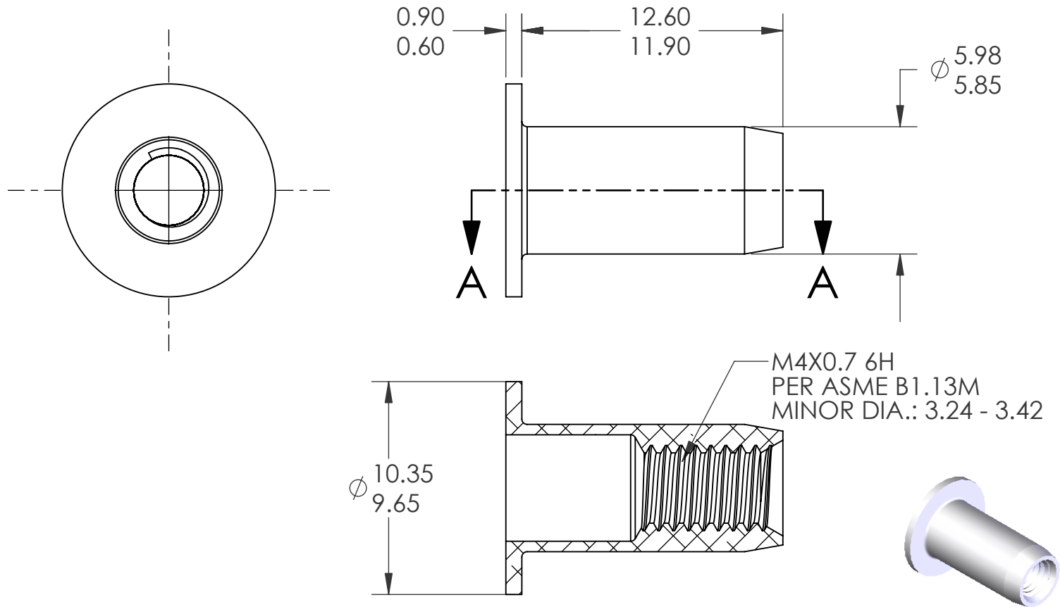
SECTION A-A
