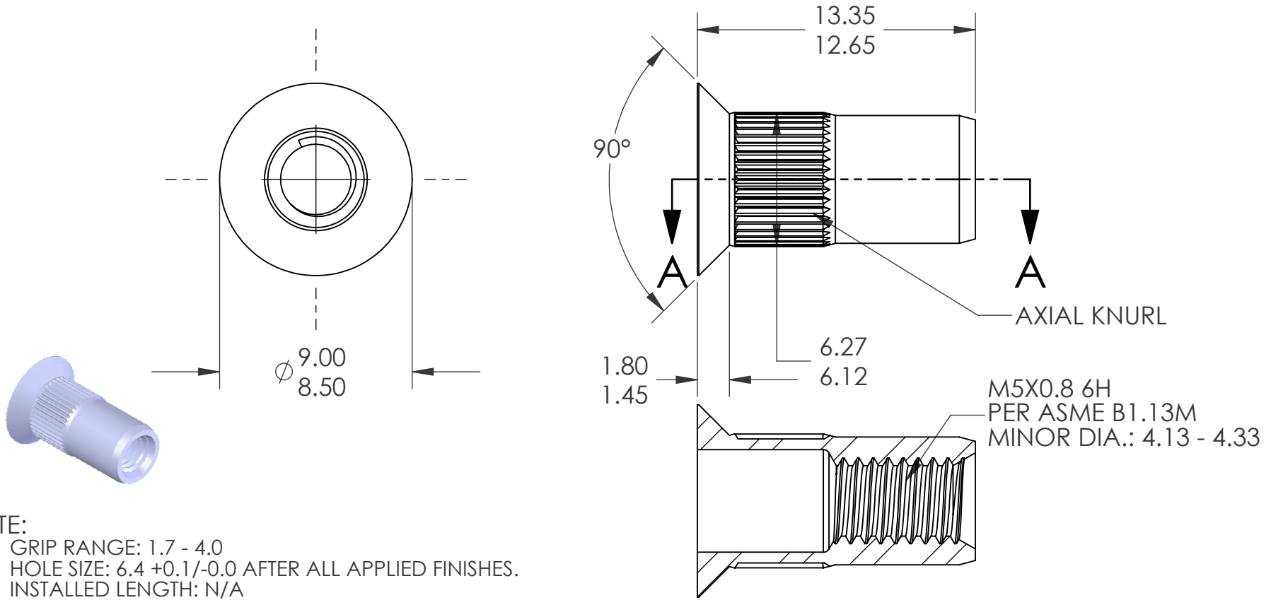
SECTION A-A
