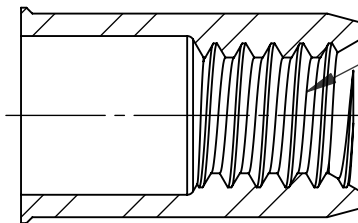
SECTION A-A SCALE 3 : 1
